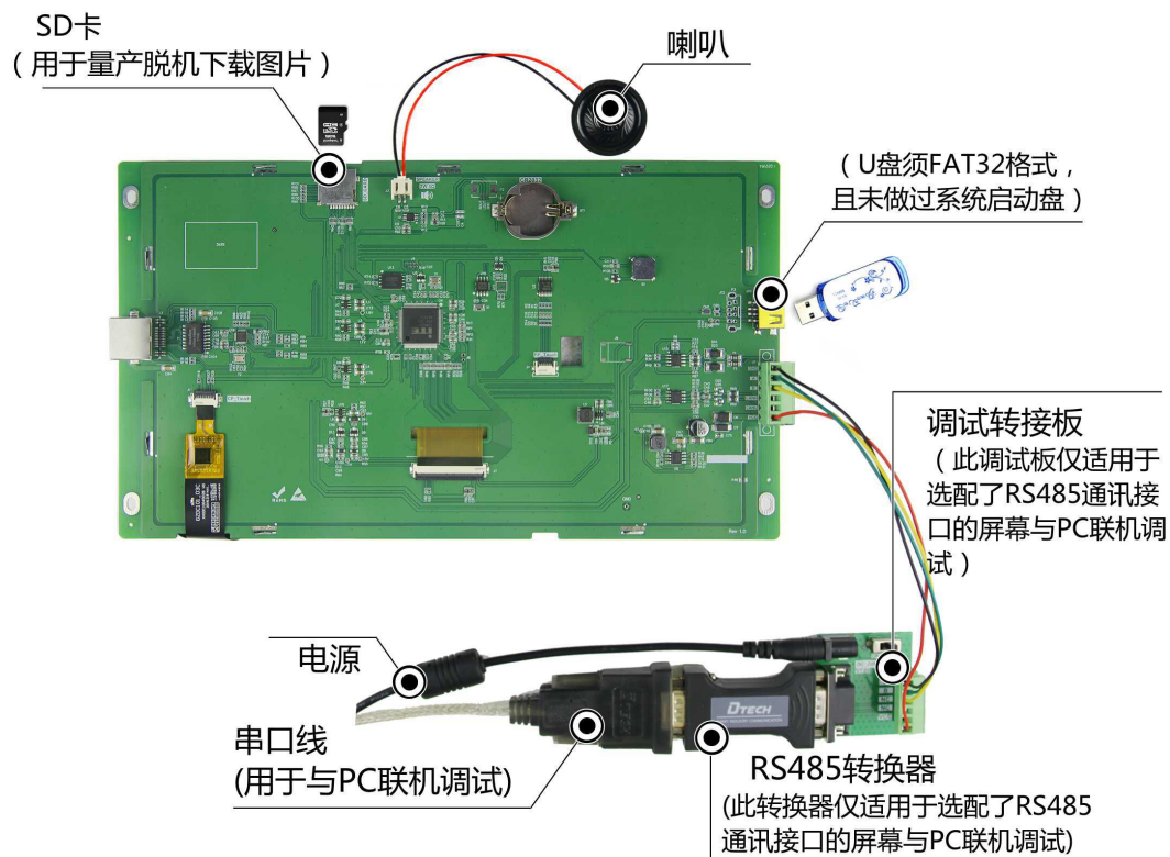
图 1-5 调试工具
