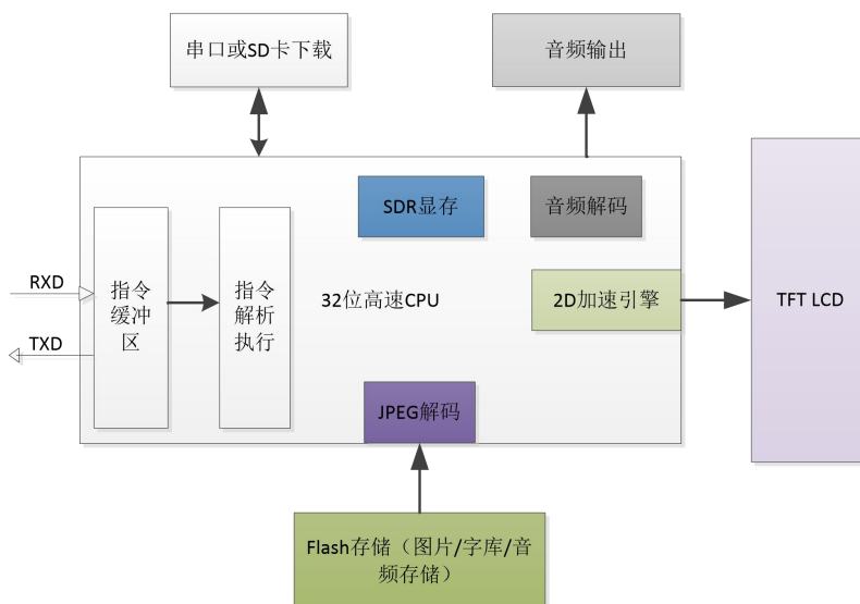
图 8-1 物联型串口屏内部结构图
