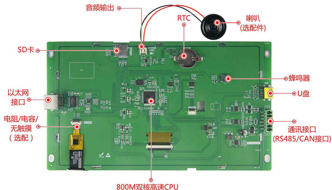
图 1-4 硬件配置图
