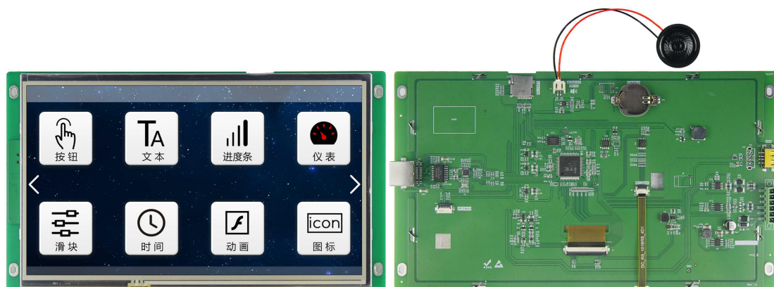
图 1-1 10.1 寸电阻触摸参考图
