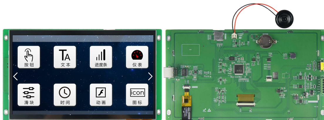
图 1-2 10.1 寸电容触摸参考图
